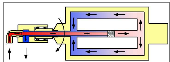
Принцип процесса с двусторонним потоком
